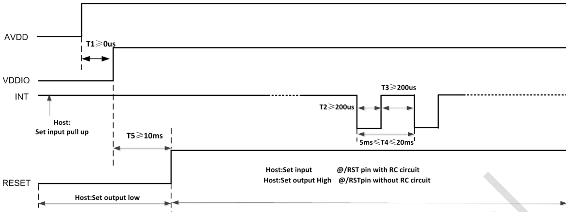
主控复位 GT917S 时序图:
