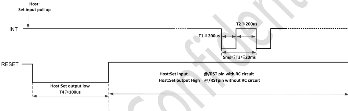
主控掉电 GT917S 时序图
