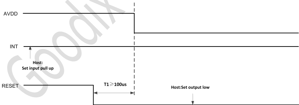
主控掉电 GT917S 时序图
